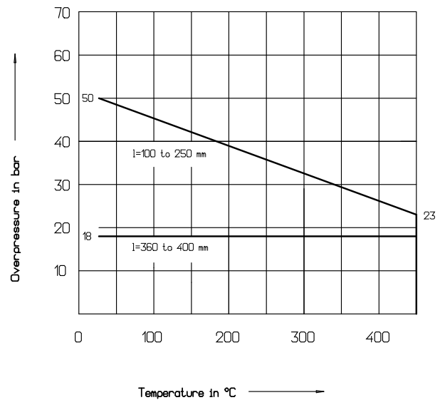
Thermowell 11 x 1mm
